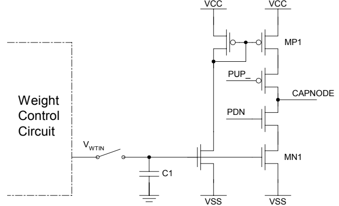
Fig.3. Synapse circuit.
