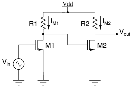
Fig. 1. Cascade amplifier.
