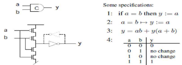
Fig. 10. The Muller C-element.
